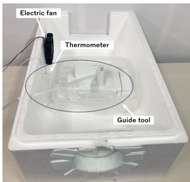
図2：恒温箱内の構造
