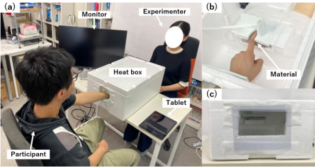
図 3 : (a) 実験の様子, (b) 参加者が実物体に触れている手元の画像, (c) 実験者側から見た恒温箱
