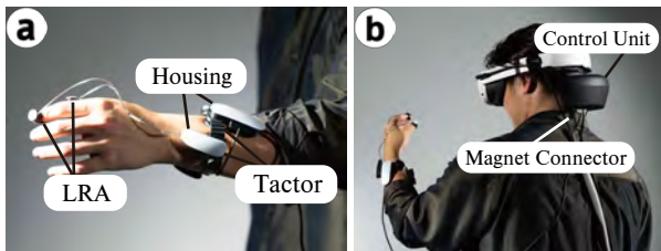
図 2: a) 手首への 4ch 回転皮膚せん断タクタと親指と人差し指の先への振動子から成る手部装着型触覚提示デバイスと b) 後頭部装着型制御ユニット。
