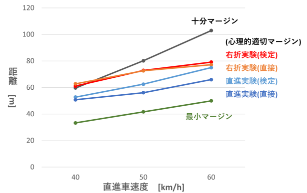
図 7: 右直マージン距離の比較
