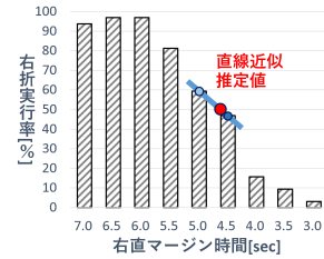
(a) 直進車 60km/h
