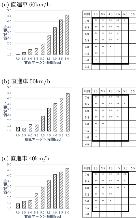
図 5: 自転車直進実験の主観評価値とパターン間有意差
