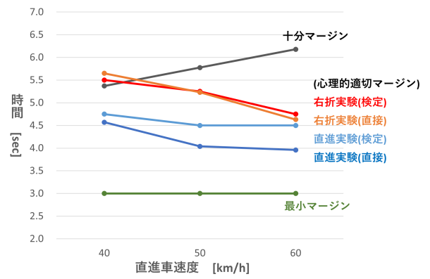
図 6: 右直マージン時間の比較
