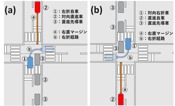
図2: 模式図, (a) 自車右折実験, (b) 自車直進実験
