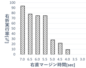
(b) 直進車 50km/h
