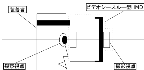
図 1: 深度ビデオスルー型 HMD における撮影視点と観察視点の不一致
