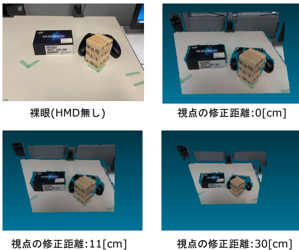
図9: 各項目における作業空間の視野
