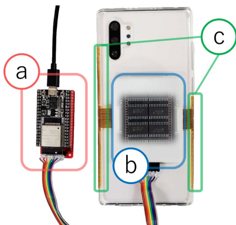
図2: 電気刺激装置 ((a): 制御部, (b): スwitching回路部, (c): 刺激提示部)
