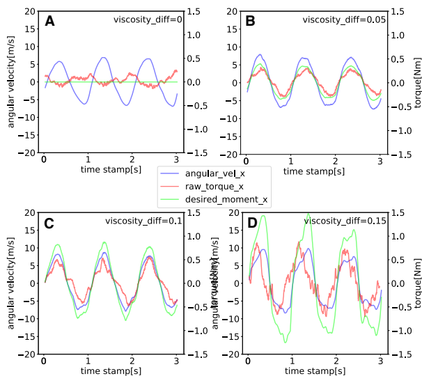
図 6: x 軸周りの 1Hz 振り動作条件における角速度 (青), 実際出力トルク (赤), 理想出力トルク \tau_D (緑). {A,B,C,D} が \Delta D_x = \{0, 0.05, 0.10, 0.15\} に対応する.
