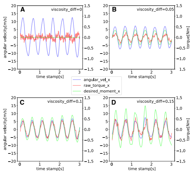
図 7: x 軸周りの振り 2Hz 動作条件における角速度 (青), 実際出力トルク (赤), 理想出力トルク \tau_D (緑). {A,B,C,D} が \Delta D_x = \{0, 0.05, 0.10, 0.15\} に対応する.
